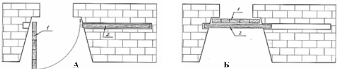
Лл. 32. Положення внутрішнього засува під час відкритого (А) та закритого (Б) дверного прорізу
