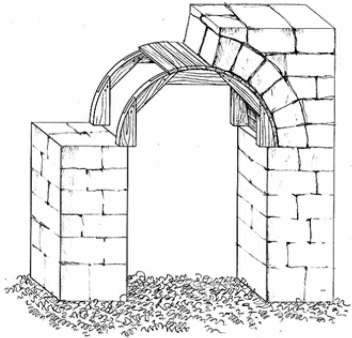
Іл. 42. Заощаджувана конструкція кружал, де замість дерев'яних стійок використані полиці в рівні п'яток арочних перемичок
