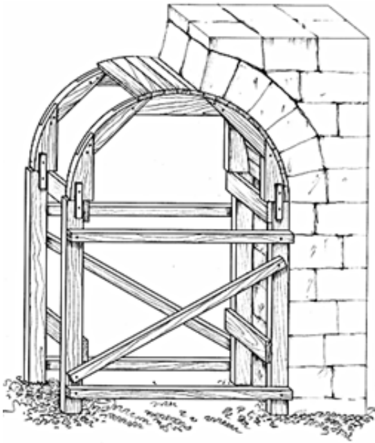
Іл. 41. Звичайна конструкція кружал для мурування арочних перемичок
