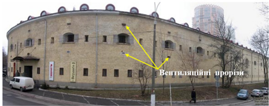
Іл. 24. Київська фортеця. Башта № 5, 1833–1846 рр. (Охор. № 867/23). Київ, вул. Печерський спуск, 16. Горизонтальні прорізи на фасаді першого та другого ярусів призначені для виходу порохових газів
