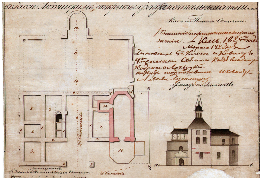
Рис. 1. План і південний фасад Десятинної церкви XVII в. в Києві на початку XIX ст. Креслення і малюнок Кіндрата Лохвицького, 1824 р. Архів Інституту археології, Національна академія наук України. Київ. Україна. Фонд 13. Справа № 9-б
