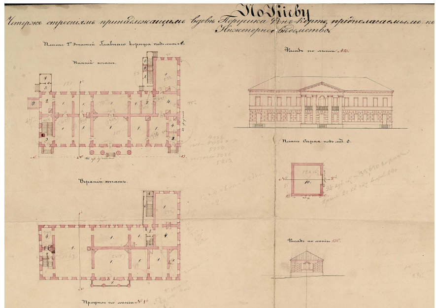
Іл. 1. Фасад і план двох поверхів будинку І. Корта 1853 р.
